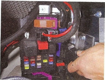
Mehr Kraft: Per Computer wird über die Service-Schnittstelle das Motor-Drehmoment angehoben. Dadurch wird auch das Schalten beeinflusst.
